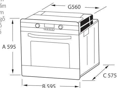
Kích thước thực sản phẩm
