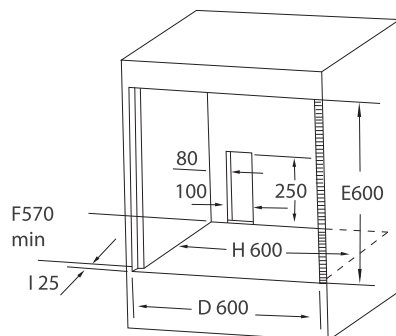
Kích thước khoét gỗ
