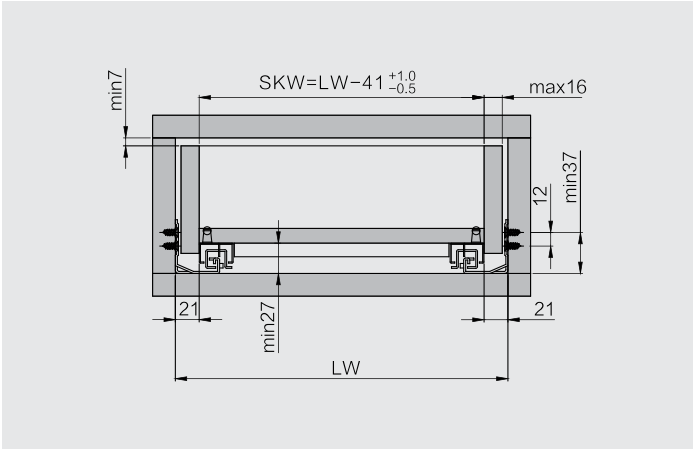
Kích thước ngăn kéo (mm)
