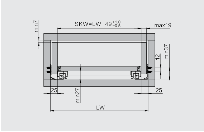
Kích thước lắp đặt (mm)
