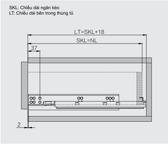
Đặc tính kỹ thuật hộp ngăn kéo (mm)
