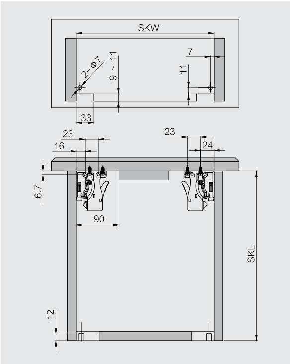
Đặc tính kỹ thuật hộp ngăn kéo (mm)
